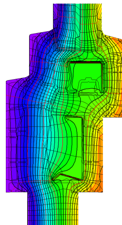
Isothermengrafik
